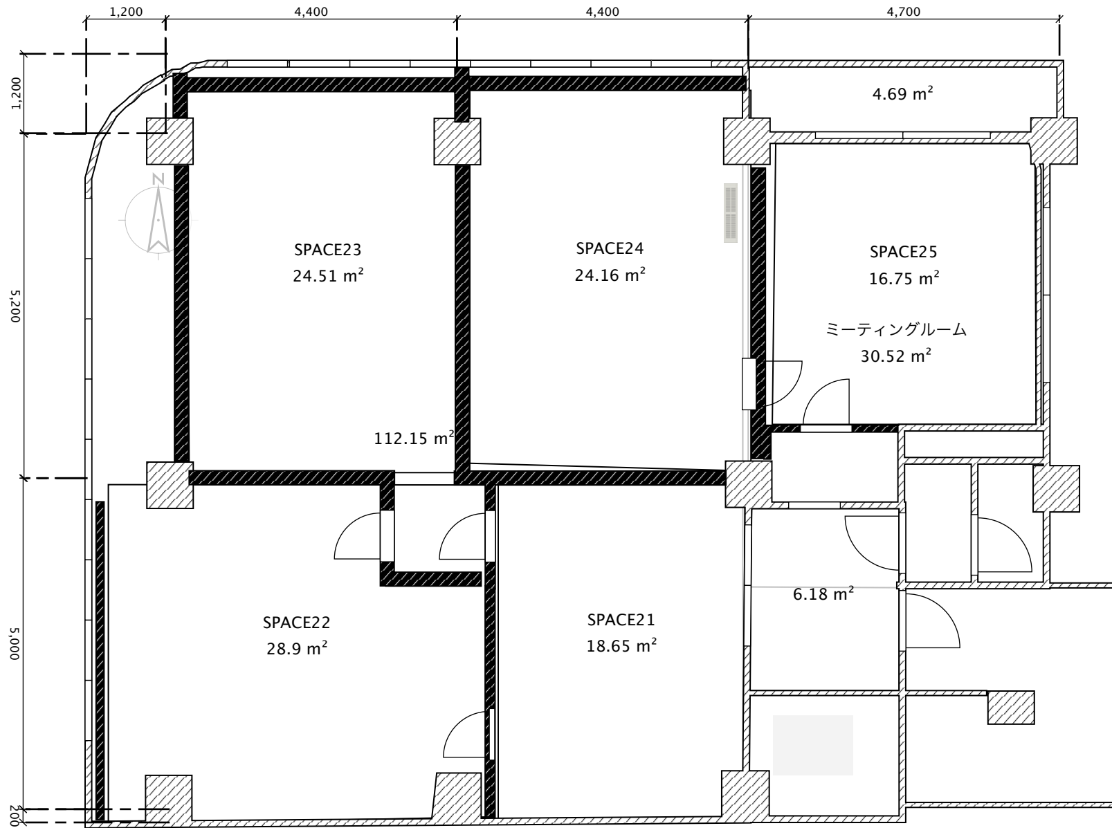
パンダスタジオ駒込（仮）2階平面図
